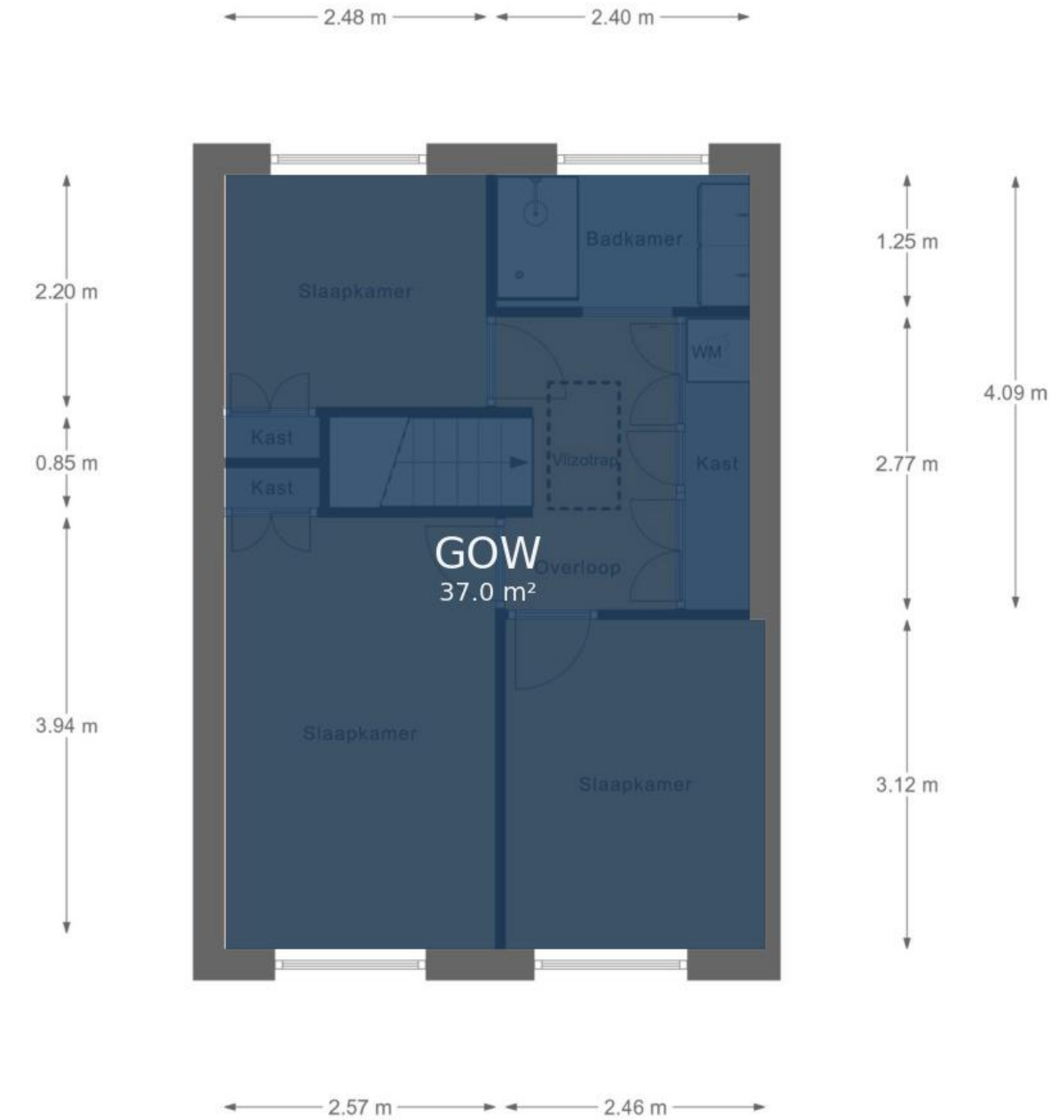
1e Verdieping
